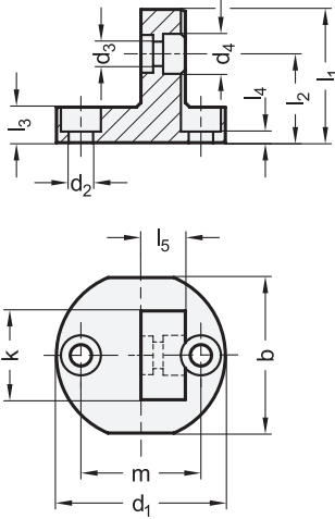
Sıkıştırma kit GN 511.1, Tip K
